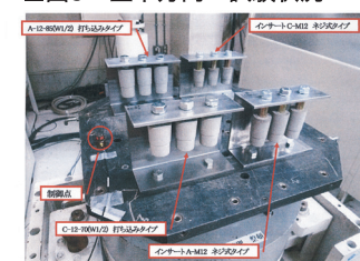
■図9 上下方向 試験状況
