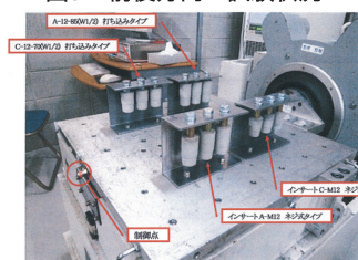
■図7 前後方向 試験状況
